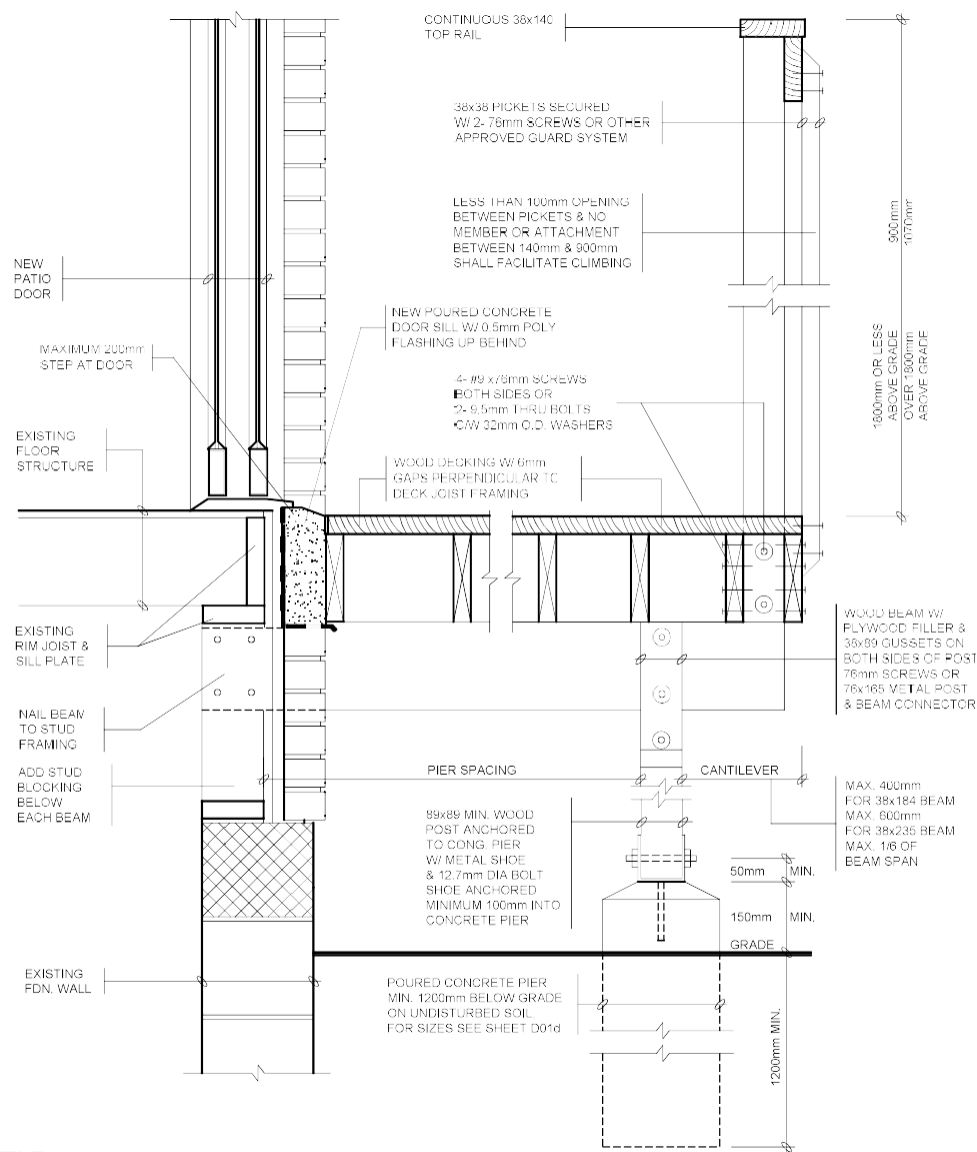
SECTION 'A'
